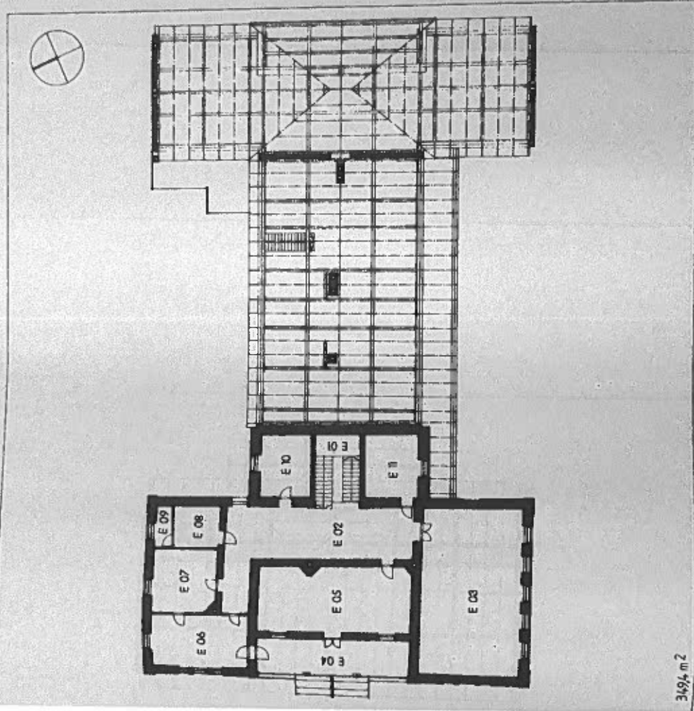
37. kép Kastély emeleti alaprajza, a terembeosztásokkal 1990.
